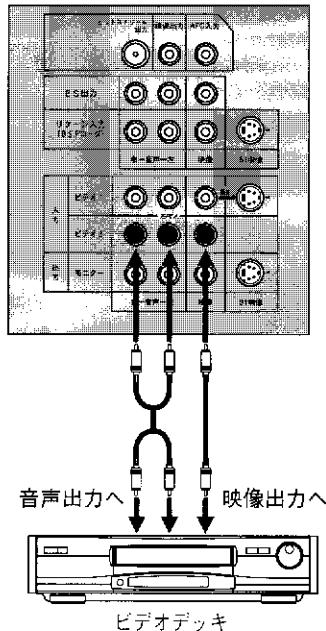
本体後面ビデオ2端子に接続する
