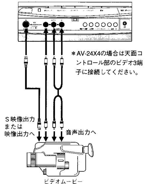
本体前面ビデオ3端子に接続する
