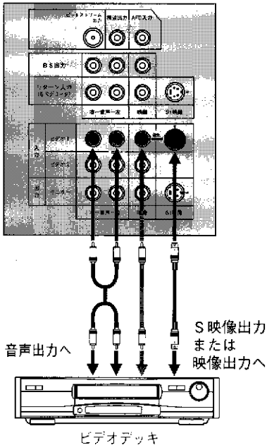
本体後面ビデオ1端子に接続する
