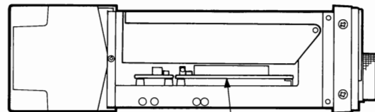
PLLユニット
