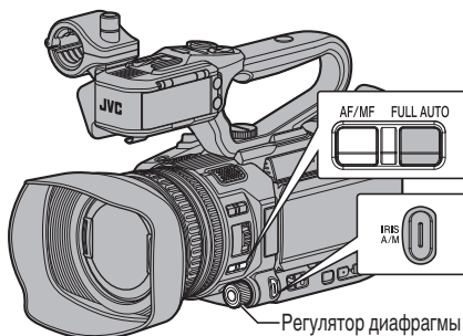
Регулятор диафрагмы
