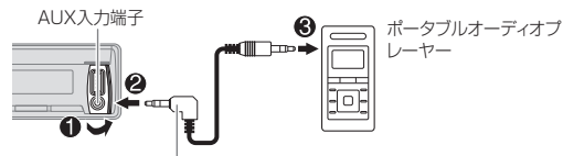
L字型コネクタのステレオミニプラグ(3.5 mm) (市販品)
