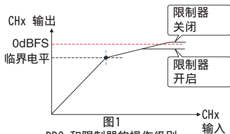
图1 DRC 和限制器的操作级别
