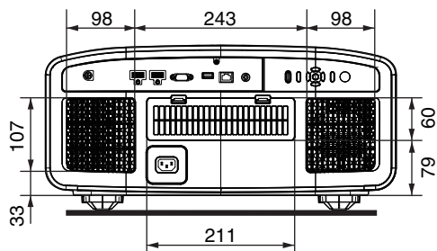
Задняя поверхность
