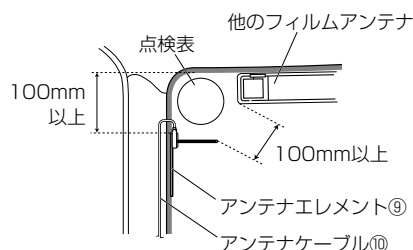
アンテナエレメントの取付方法
