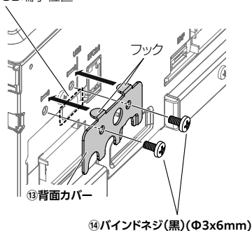
⑭バインドネジ(黒)(Φ3x6mm)
