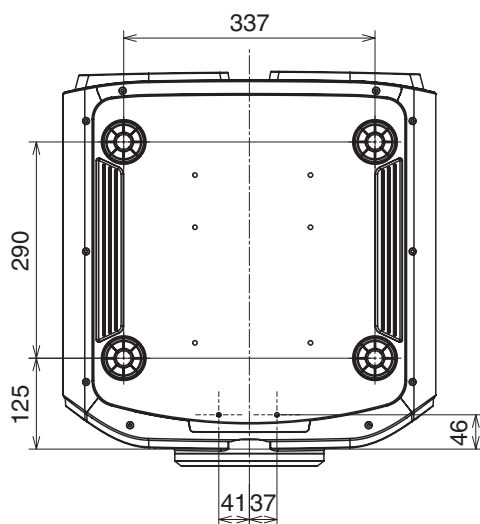
Unterseite
