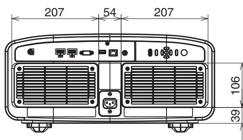
Rückseite
