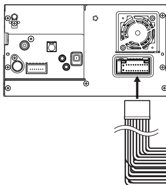
電源ハーネス③
