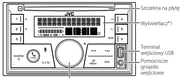
Pokrętko głośności
