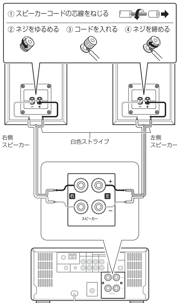
スピーカー端子 (アンプまたはレシーバー)
