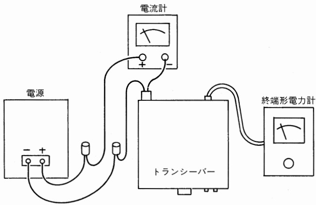
[接続例]
