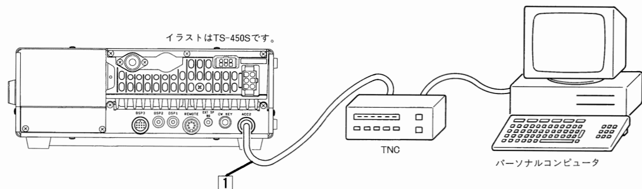
ACC2コネクター接続図
