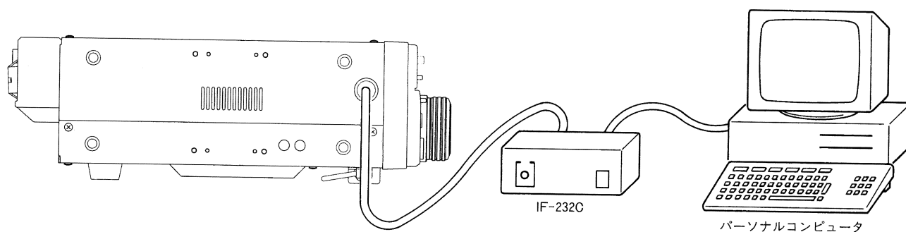
接続図
