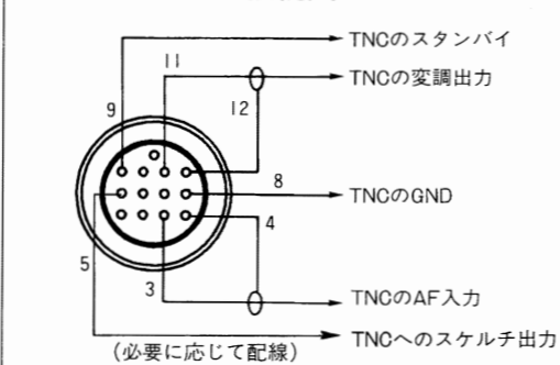
ACC2コネクター接続図
