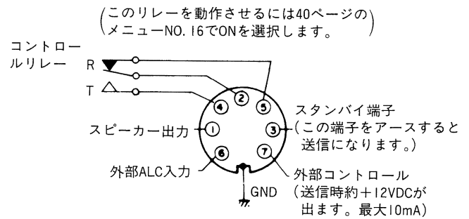
セットの後方より見た図
