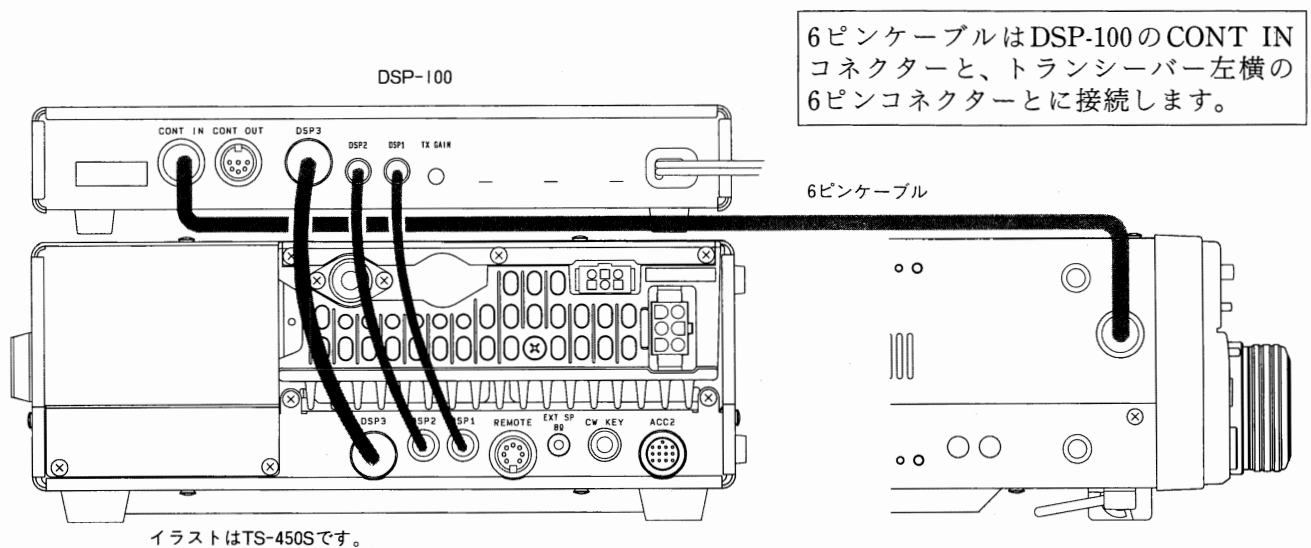
接続図
