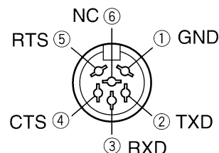
TS-450S/690S/850S/ 950SDX の ACC 1 背面パネルから見たところ
