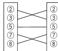
COM 端子と配線
