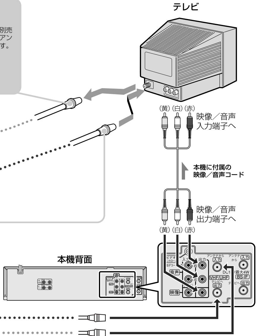
75Ω同軸ケーブル（プラグ付き）
