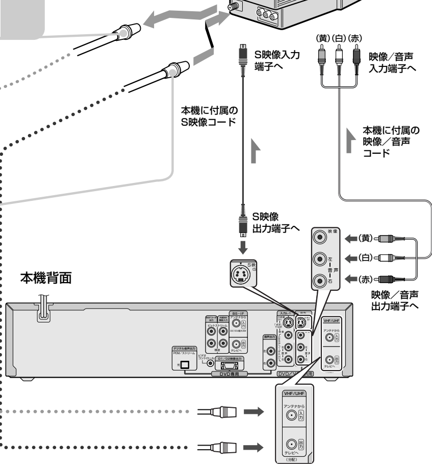
75Ω同軸ケーブル（プラグ付き）
