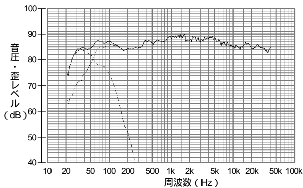
中型フロアタイプスピーカー + SX-DW7 CUT OFF SELECTOR 40 Hz
